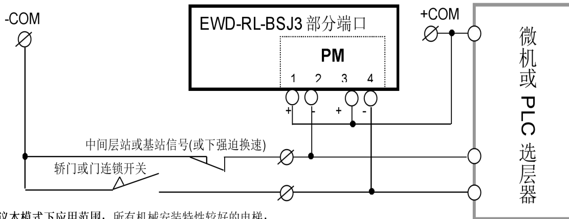
附图：PM 端口，自适应模糊层站补偿接线方式
